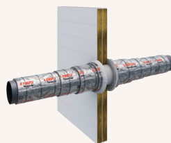
V153 | -/240/240
