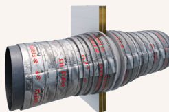
V151 | -/240/240
